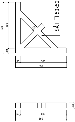
CHI TIẾT SONCON TL: 1/15
